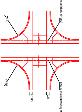
DETALLE DE JUNTAS DE BOCA CALE PARA CORDON CUENTA DE H° (proyectado)
